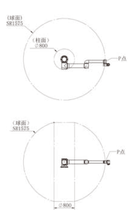
AUBO-iS25(Ex) 本体P点运动范围
