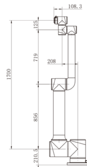
AUBO-iS25(Ex) 外形尺寸图
