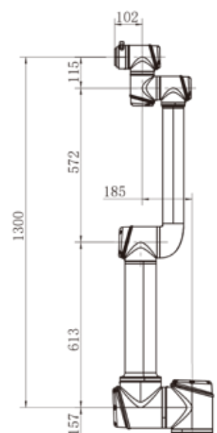
AUBO-iS10(Ex) 外形尺寸图
