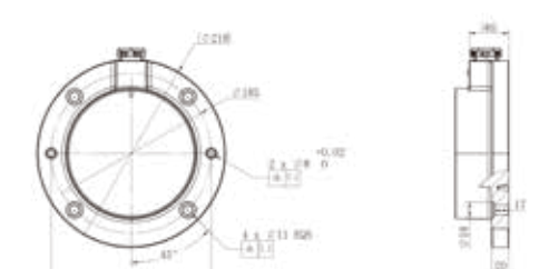
AUBO-iS10(Ex) 基座俯视图
