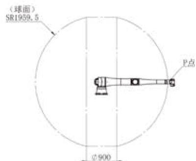
AUBO-iS35(Ex) 本体P点运动范围
