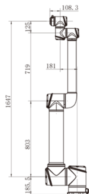
AUBO-iS20(Ex) 外形尺寸图
