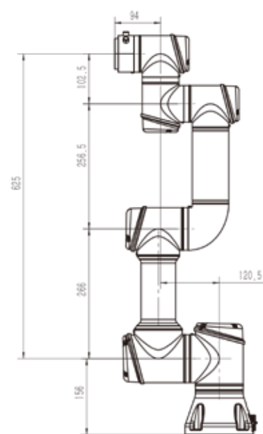
AUBO-iS3(Ex) 外形尺寸图
