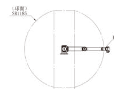
AUBO-iS10(Ex) 本体P点运动范围
