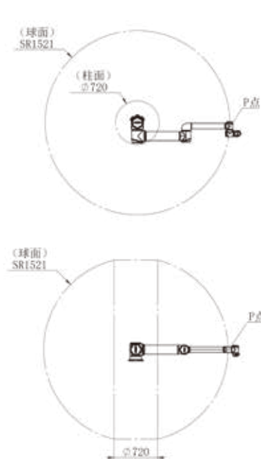
AUBO-iS20(Ex) 本体P点运动范围
