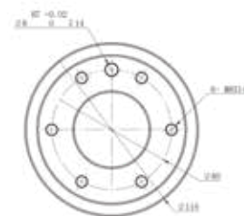
AUBO-iS35(Ex) 末端法兰
