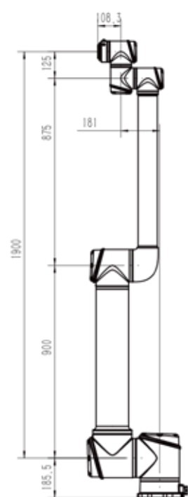
AUBO-iS16(Ex) 外形尺寸图
