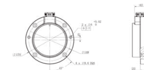
AUBO-iS7(Ex) 末端法兰
