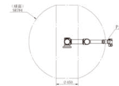
AUBO-iS7(Ex) 本体P点运动范围
