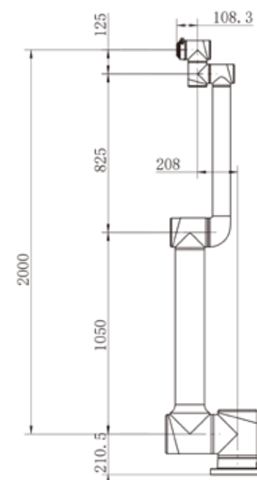
AUBO-iS20L(Ex) 外形尺寸图
