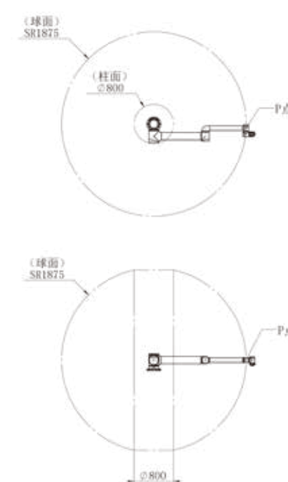
AUBO-iS20L(Ex) 本体P点运动范围
