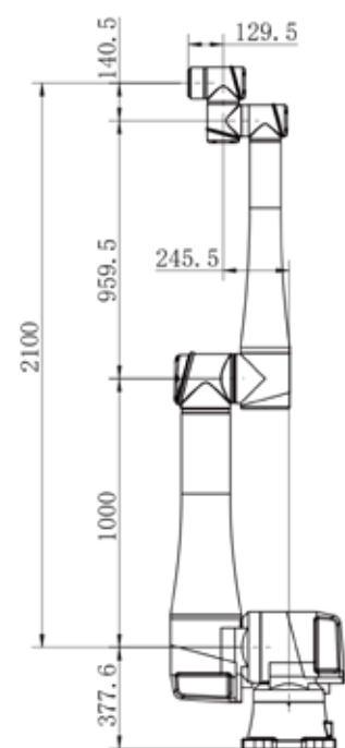
AUBO-iS35(Ex) 外形尺寸图
