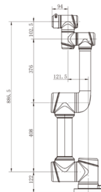
AUBO-iS7(Ex) 外形尺寸图
