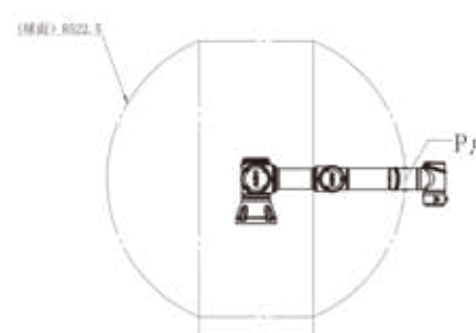
AUBO-iS3(Ex) 本体P点运动范围
