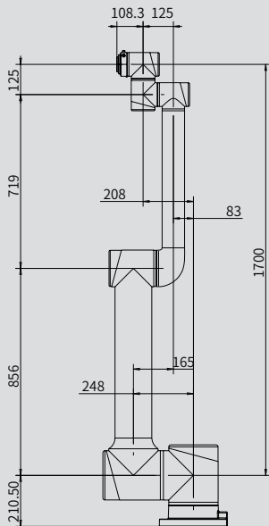
AUBO-iS25 外形尺寸图
