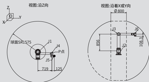
AUBO-iS25 本体P点运动范围
