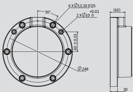
AUBO-iS25 基座俯视图
