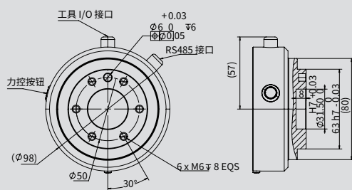
AUBO-iS25 末端法兰
