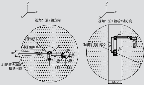
AUBO-iS20 本体P点运动范围
