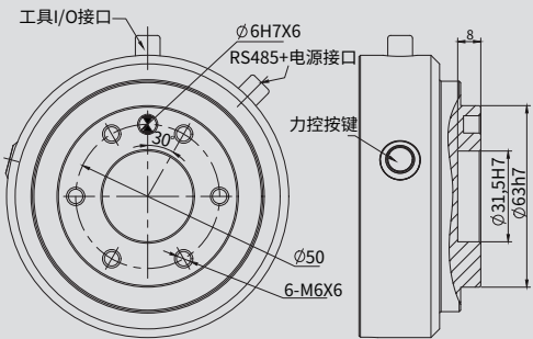
AUBO-iS20 末端法兰
