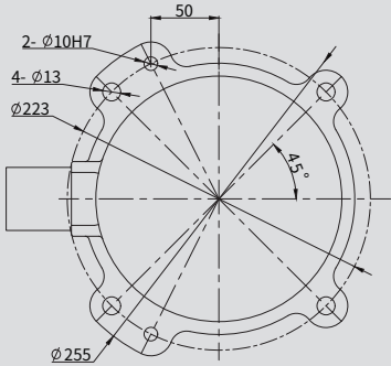
AUBO-iS20 底座俯视图
