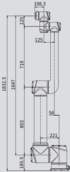
AUBO-iS20 外形尺寸图
