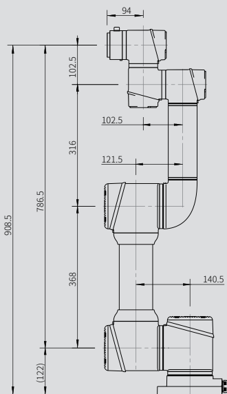
AUBO-i7H 外形尺寸图
