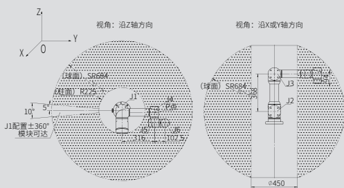
AUBO-i7H 本体P点运动范围
