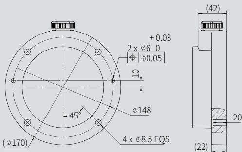
AUBO-i7H 末端法兰
