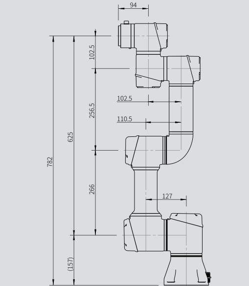
AUBO-i3H 外形尺寸图
