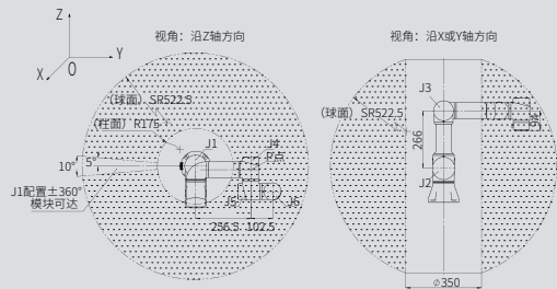
AUBO-i3H 本体P点运动范围
