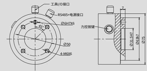
AUBO-i3H 末端法兰
