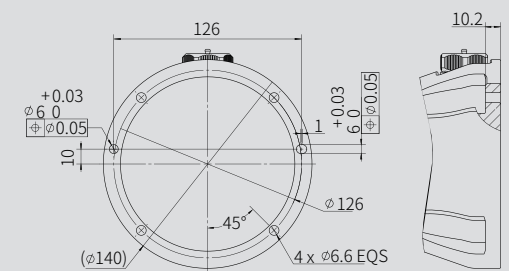
AUBO-i3H 基座俯视图
