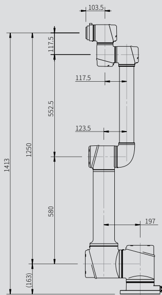
AUBO-i12H 外形尺寸图
