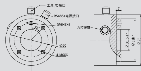
AUBO-i12H 末端法兰
