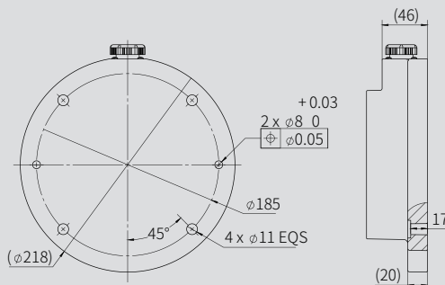
AUBO-i12H 基座俯视图
