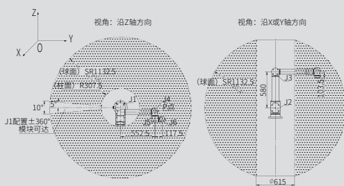
AUBO-i12H 本体P点运动范围
