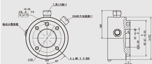
AUBO-i7 末端法兰
