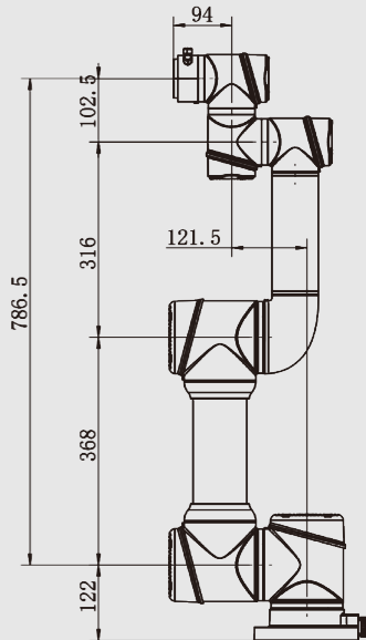
AUBO-i7 外形尺寸图
