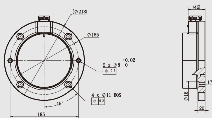
AUBO-i10 基座俯视图
