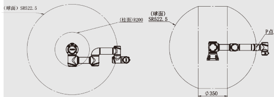
AUBO-i3 本体P点运动范围
