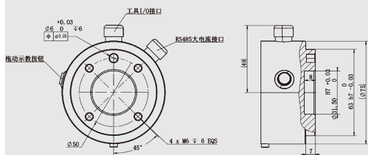
AUBO-i10 末端法兰
