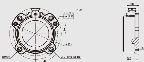
AUBO-i20 基座俯视图
