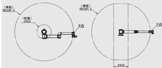
AUBO-i10 本体P点运动范围
