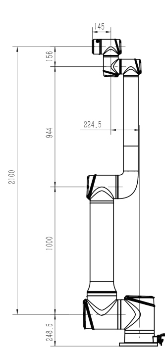
AUBO-G35 外形尺寸图
