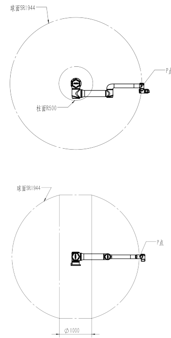
AUBO-G35 本体P点运动范围
